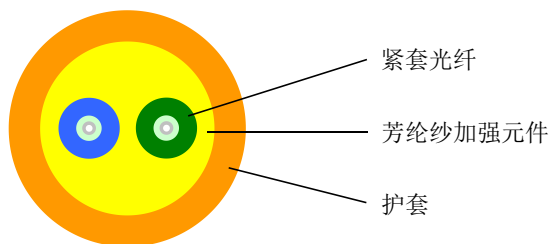
双芯圆形室内光缆 I 型
